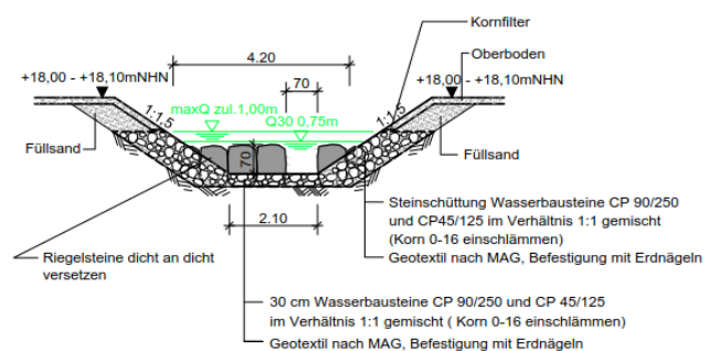
Regelquerschnitt - Umgehungsgerinne M 1:100
